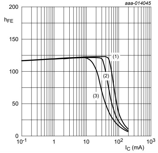
T_{amb} = 25\text{ }^\circ\text{C} (1) V_{CE} = 50\text{ V} (2) V_{CE} = 25\text{ V} (3) V_{CE} = 10\text{ V}
